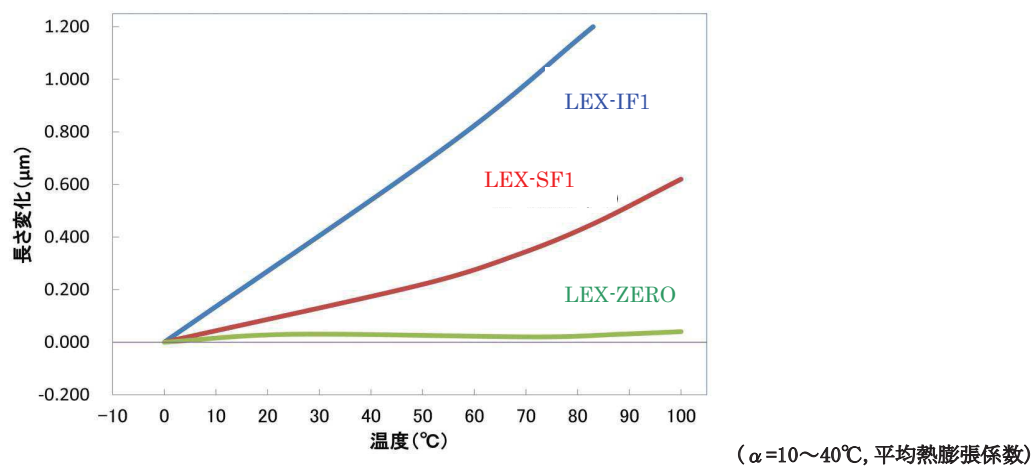
図2 当社低熱膨張材との熱膨張曲線の比較
